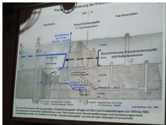
Geologische Schnittdarstellung, der Entwässerungssysteme
